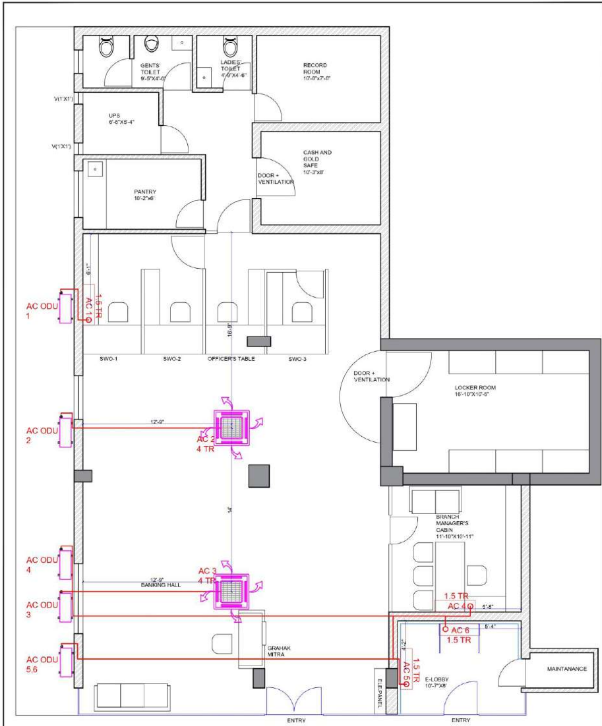
A.C. LAYOUT
